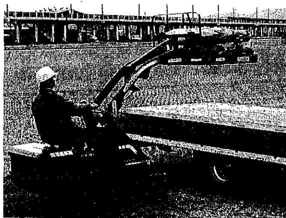
乗用ローダによる4トントラックへの積み込み作業
