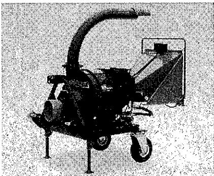
農用トラクタ装着の「GF170TR」
