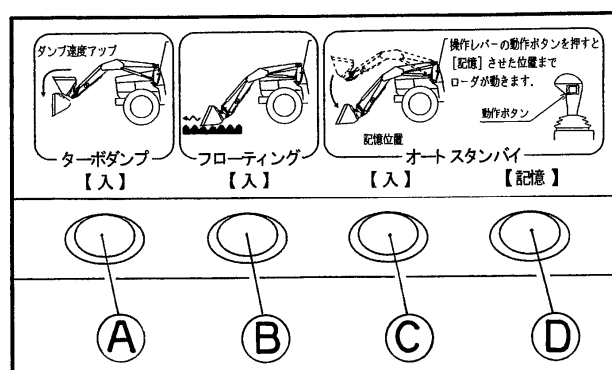
操作パネル
