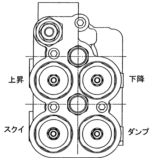
バルブ側ソレノイド部
