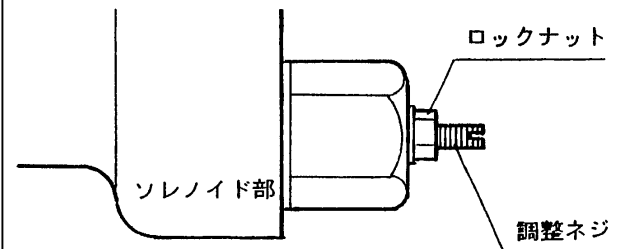
調整部詳細
