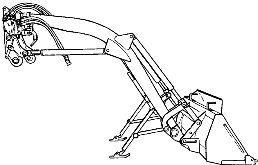
▲ 上図は電磁弁式ローダーの場合
