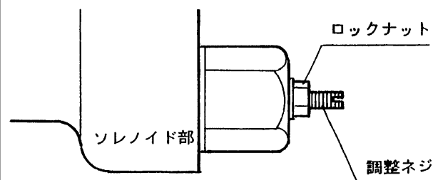
調整部詳細
