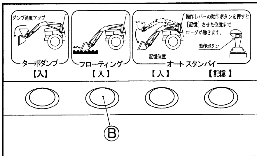
操作パネル（右図）
