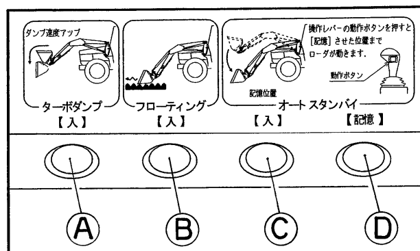
操作パネル
