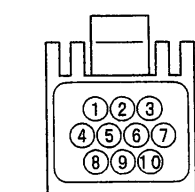
(A)から見た図 (10 極コネクタ裏側)
