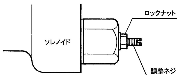
ソレノイド調整部詳細
