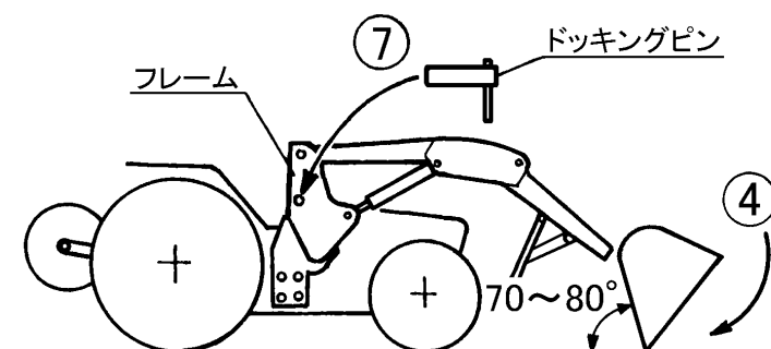
電磁弁ローダの場合
