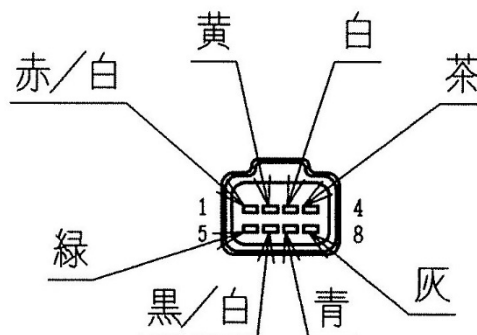
8 極コネクタ (①から見た図)
