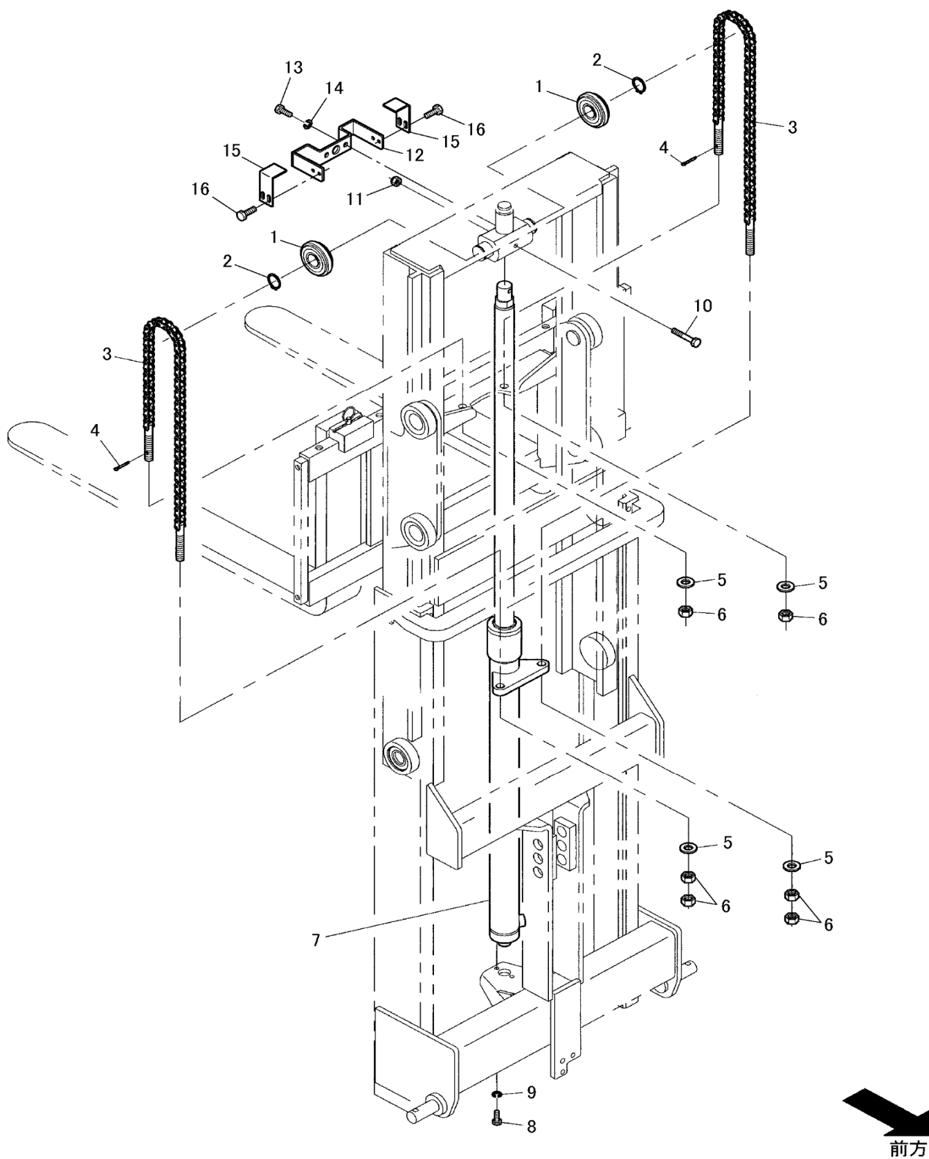
FIG.3 チェーン部
