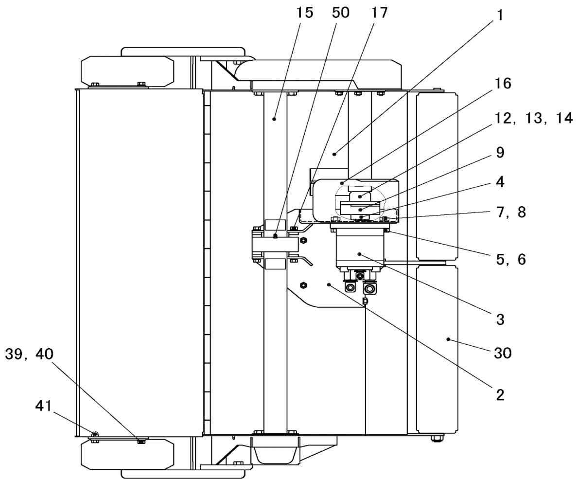
FIG.2 モアー詳細(2)
