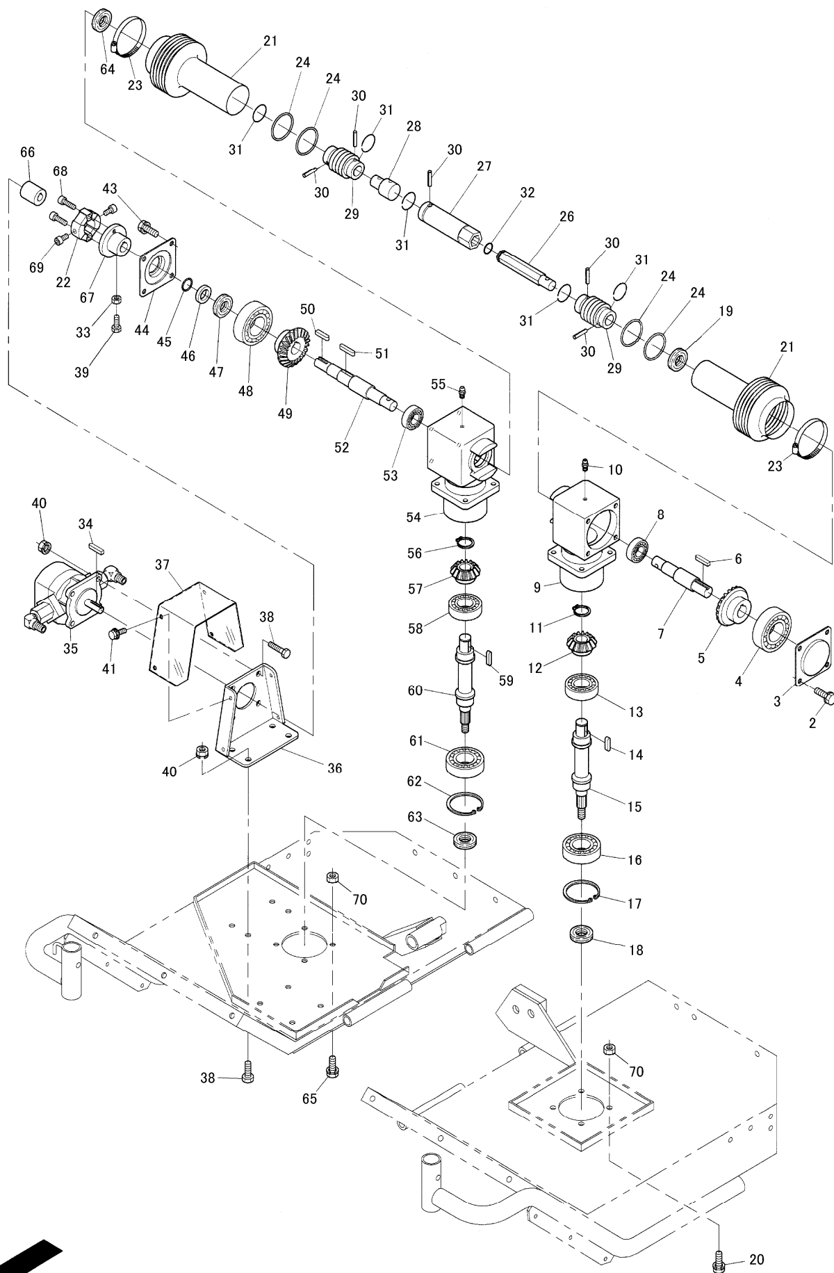
FIG.3 モアー詳細(3)
