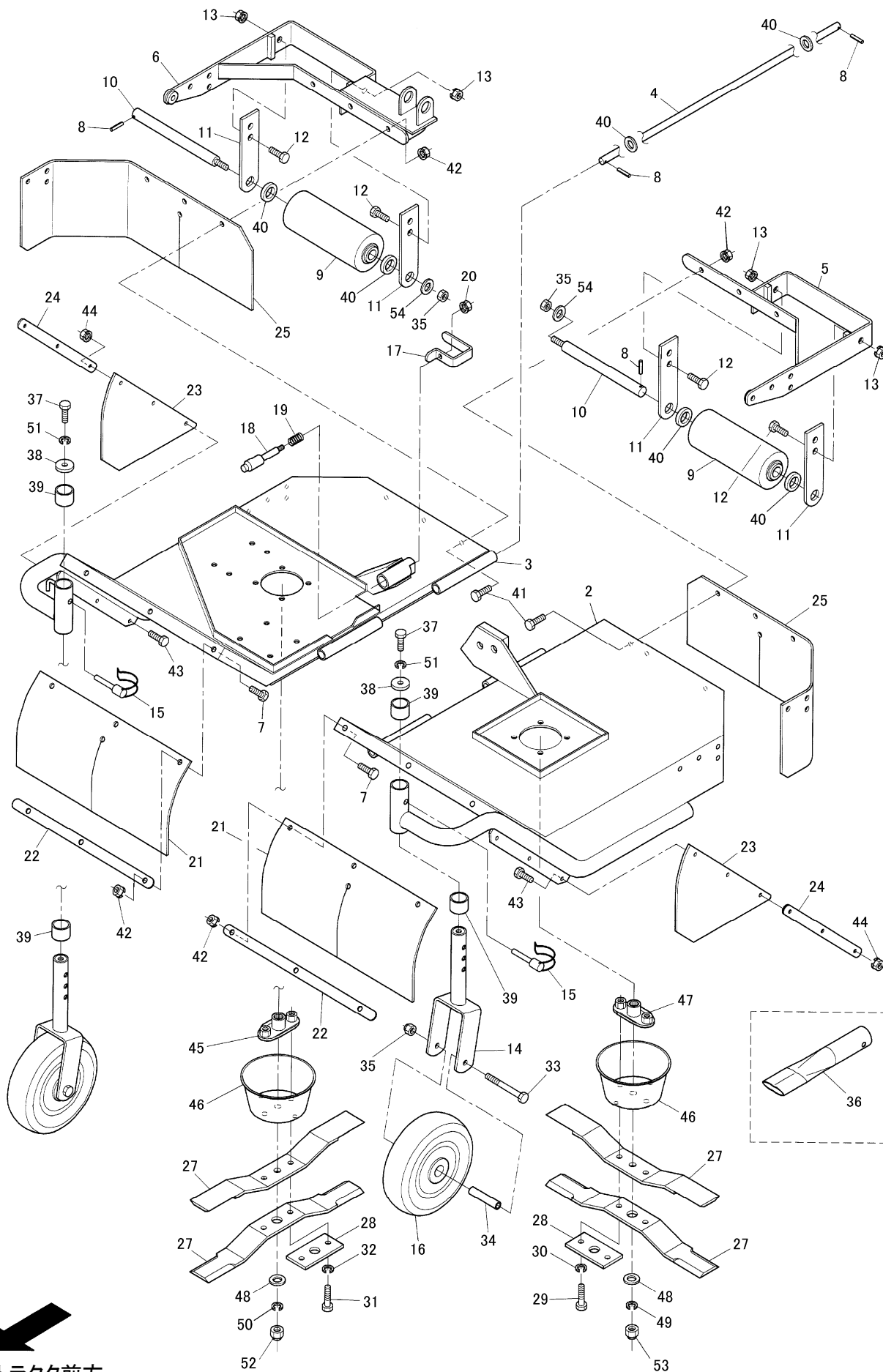
FIG.1 モアー詳細(1)
