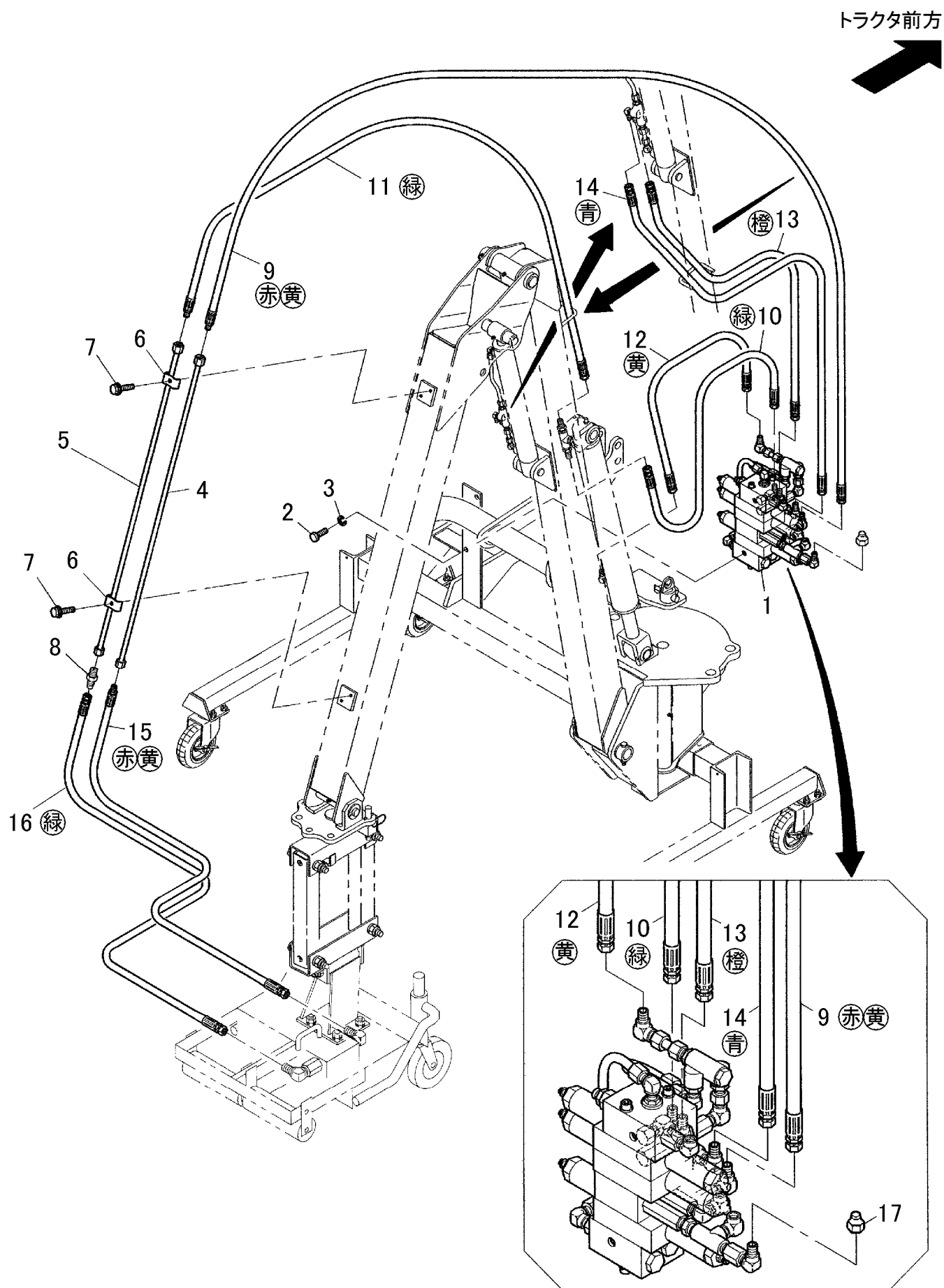
FIG.3 アーム配管
