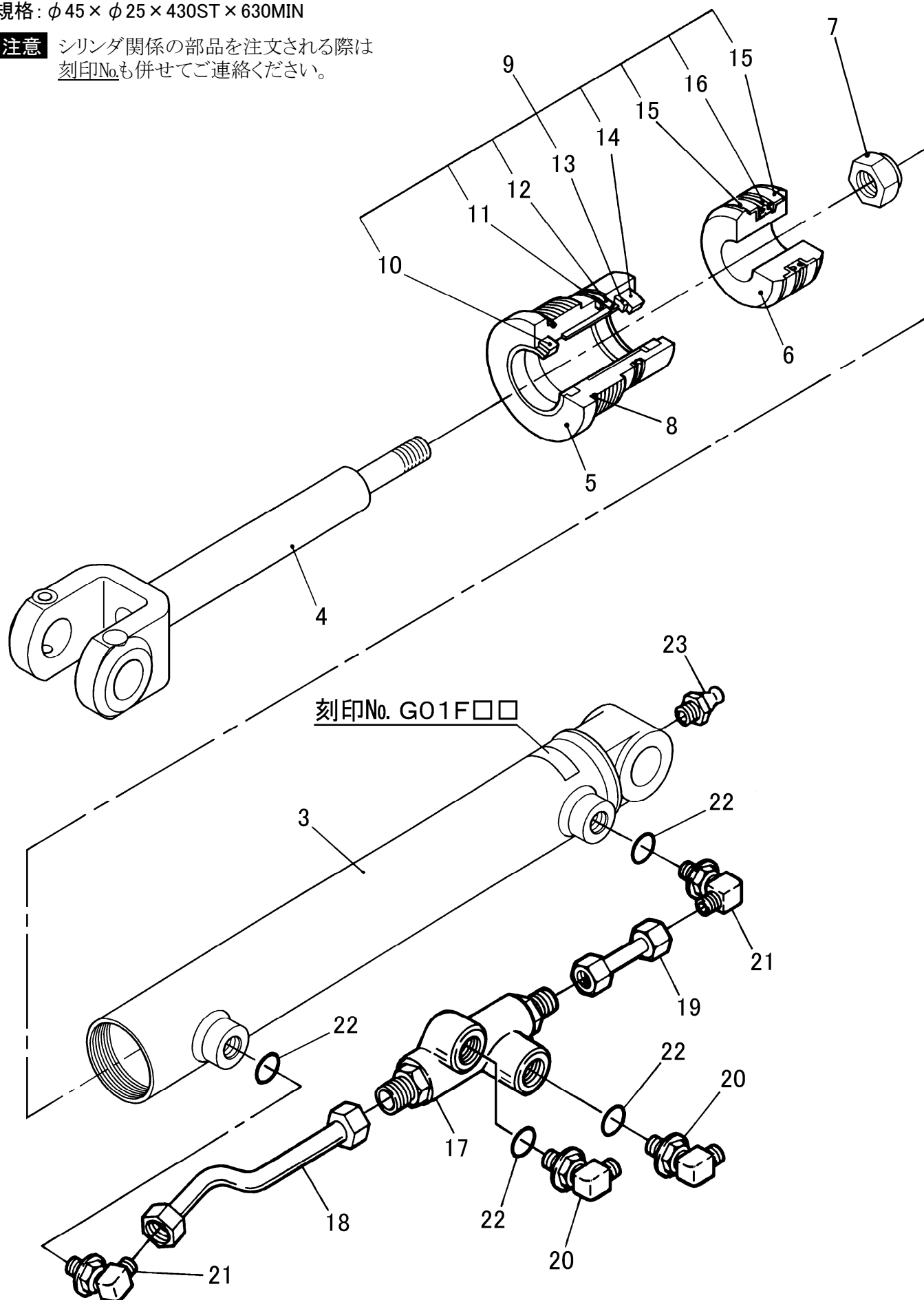
FIG.5 シリンダ2詳細
