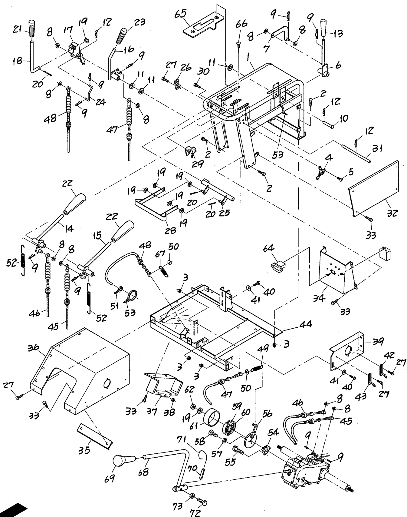
FIG.5 コントロールボックス(1)
