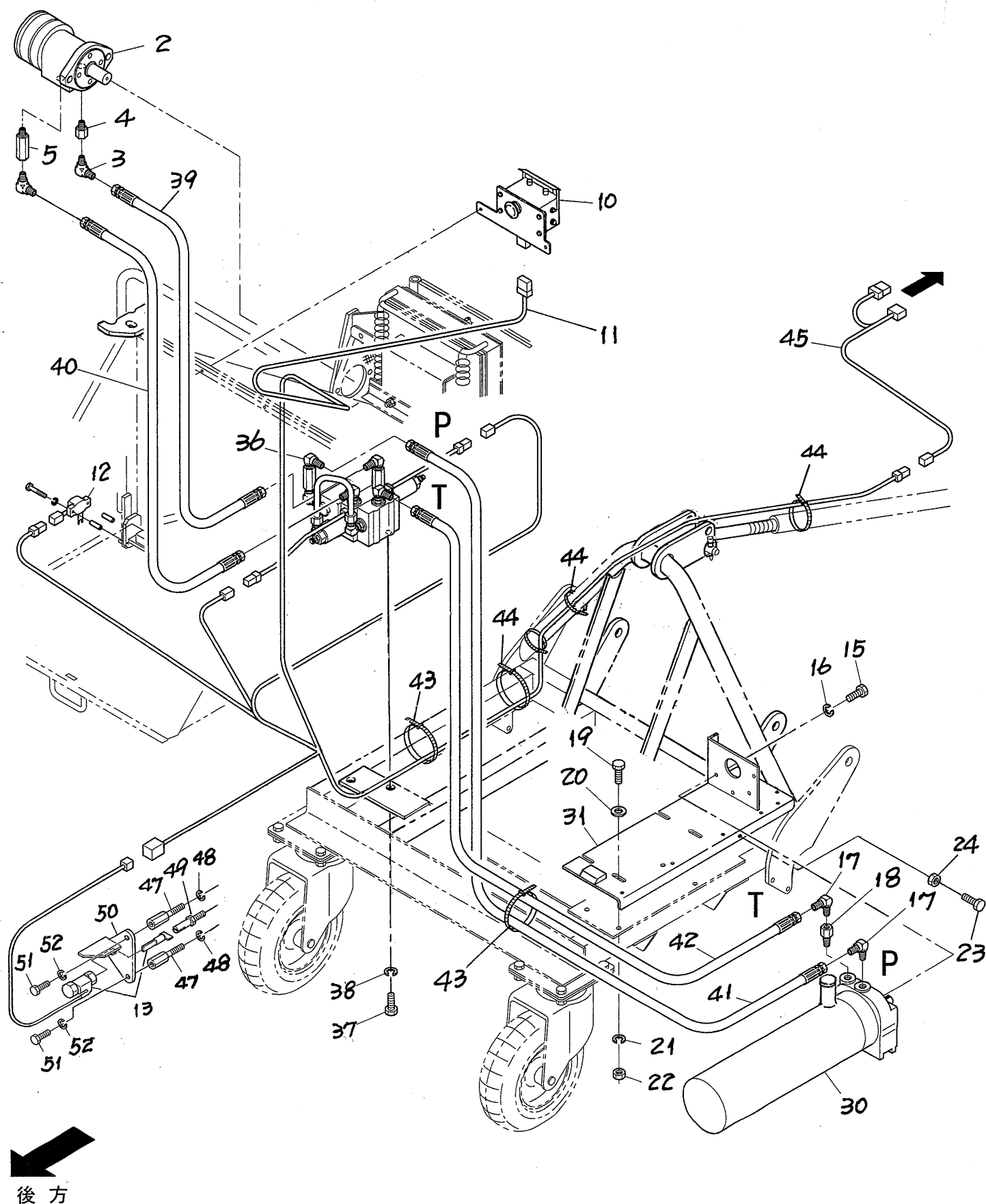
FIG.8 油圧・電気システム(2)
