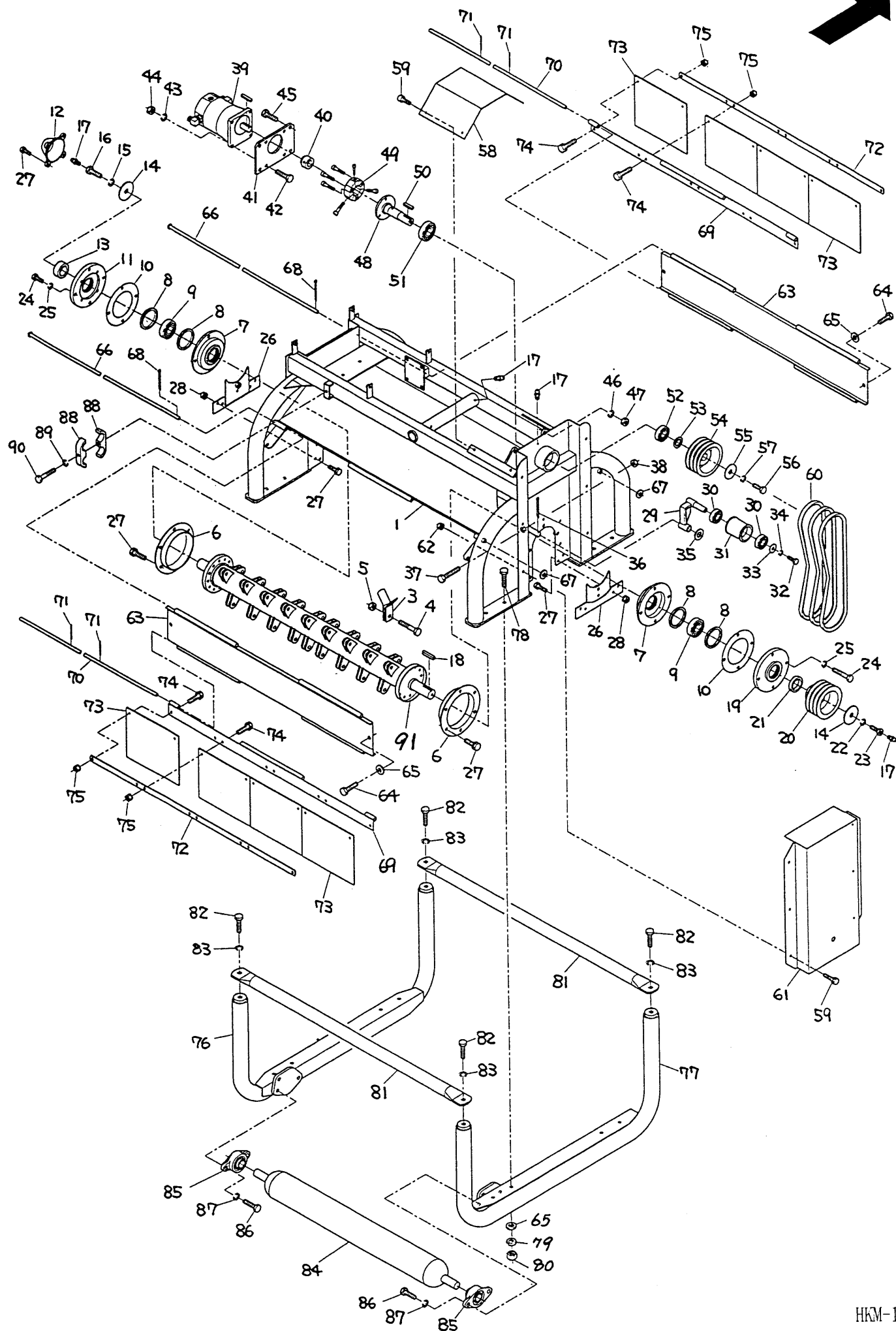
FIG. 3 モーター本体詳細 (2)
