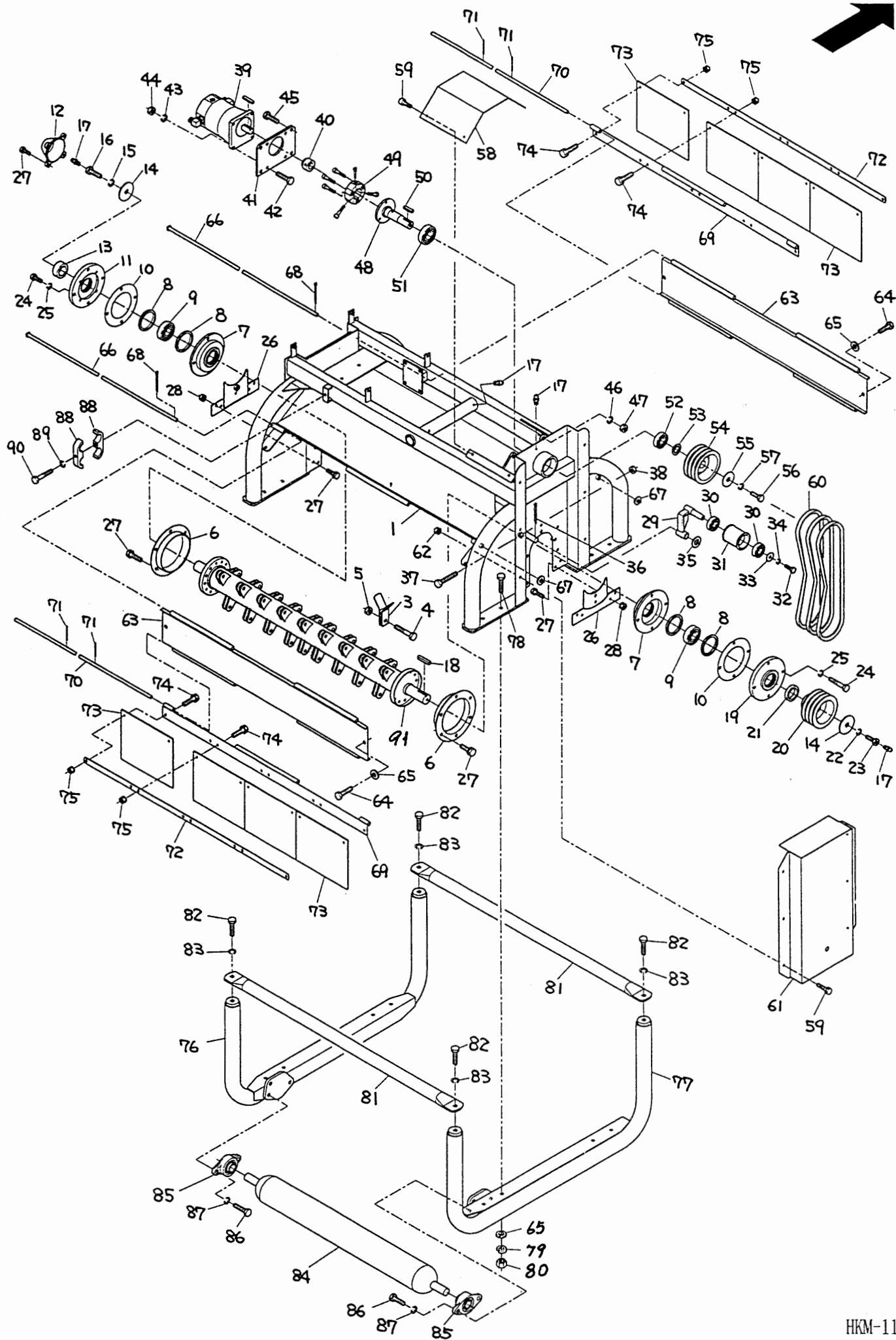
FIG. 2 モア一本体詳細 (1)
