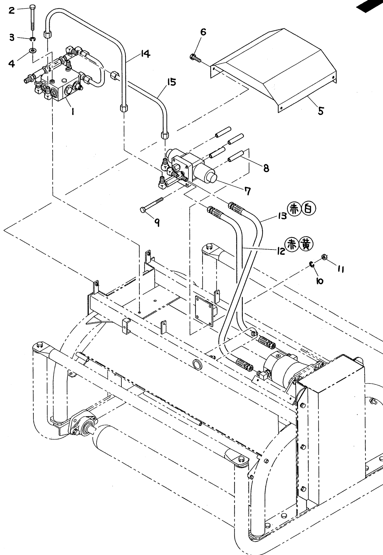
FIG. 5 バルブ配管 (D×仕様の場合)
