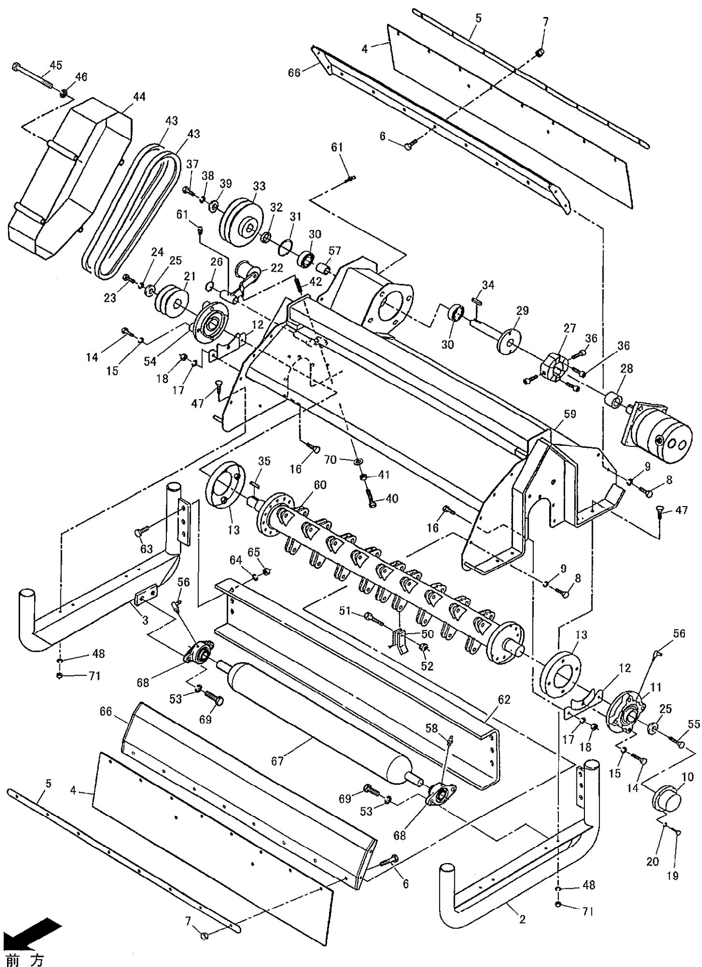
FIG.4 モア一本体詳細(1)
