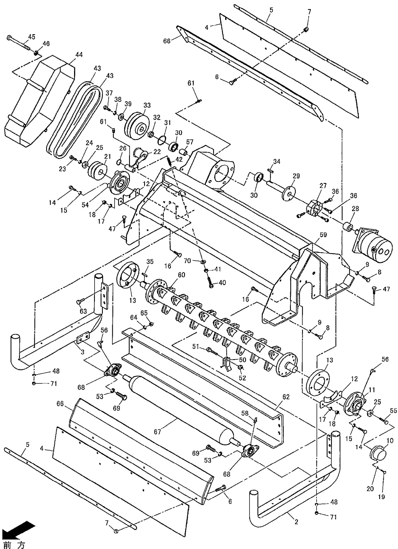
FIG.5 モア一本体詳細(2)
